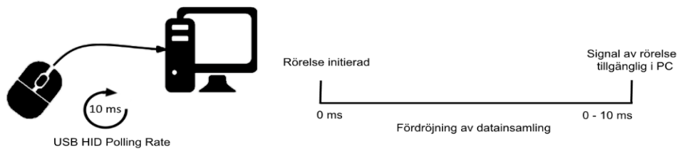
Figur 1: Normal tidsförskjutning av USB mus
